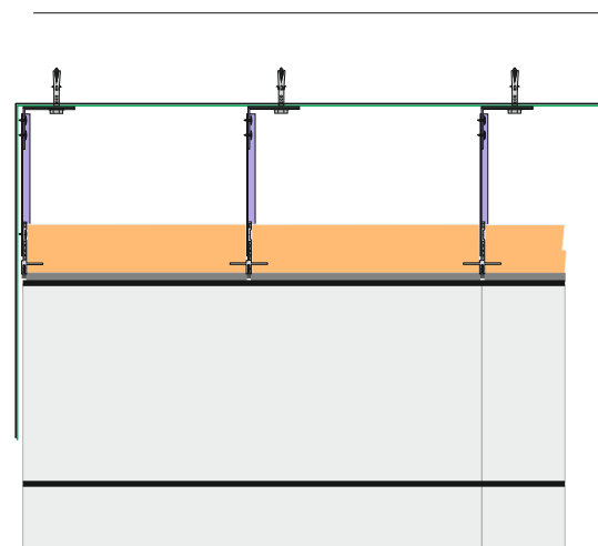
SECCIÓN FRONTAL
