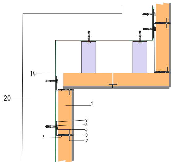
SECCIÓN TRANSVERSAL
